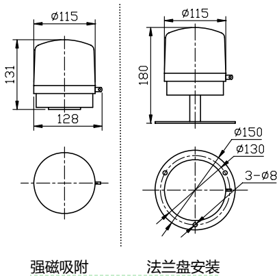
安装尺寸图 (单位: mm)
