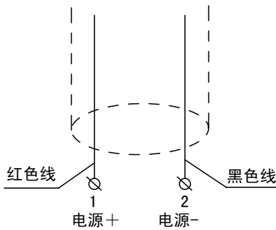
接线示意图
